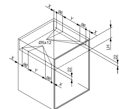
前板加工図
