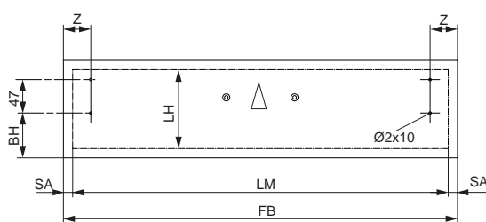
前板加工図
